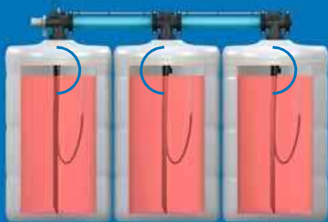
Czujnik maksymalnego napełnienia w każdym zbiorniku oraz pływający króciec pobierania
